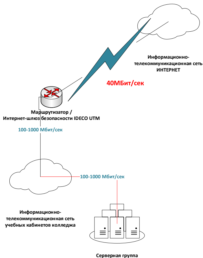
Структурная схема аппаратной части ЕИОС ГБПОУ ВО «ВГППК»
